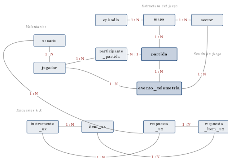
Figura 1: Diagrama Entidad-Relación conceptual. Las cardinalidades se muestran en rojo sobre cada relación; los hubs centrales del modelo ( partida y evento_telemetria ) aparecen en color más intenso.
